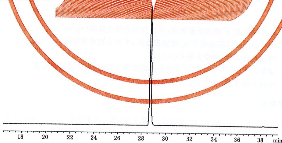
图 E.1 苯并[a]芘参考色谱图
